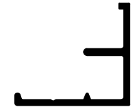
Alüminyum Başlangıç Profili 20x23 mm
