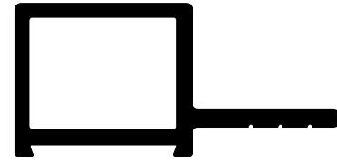
Bitiş Modülü 26x30 mm
